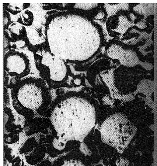
Fig. 6. Akrylatyta efter borstning med Ultra-Weiss (12 tim). Skala 112:1. Enligt Meiners 1973.
