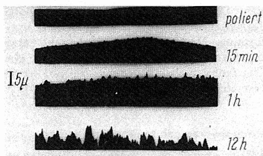
Fig. 4. Akrylatyta efter borstning med Ultra-Weiss (15 min, 1 tim, 12 tim). Enligt Meiners 1973.
