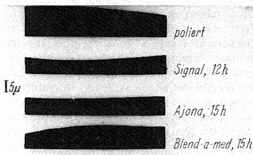
Fig. 5. Akrylatyta efter borstning med Signal (12 tim), Ajona (15 tim) och Blend-a-med (15 tim). Enligt Meiners 1973.
