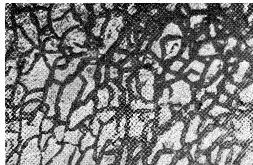
Fig 3. Fasadakrylat polymeriserat under tryck exponerat för kloroform under 30 sekunder. (Bilden tagen med 50 gångers förstoring med påfallande ljus.) Man ser tydligt att den lägre polymeriserade vätskan lösts ut, medan kornen fortfarande står kvar och bildar nätmönster.
